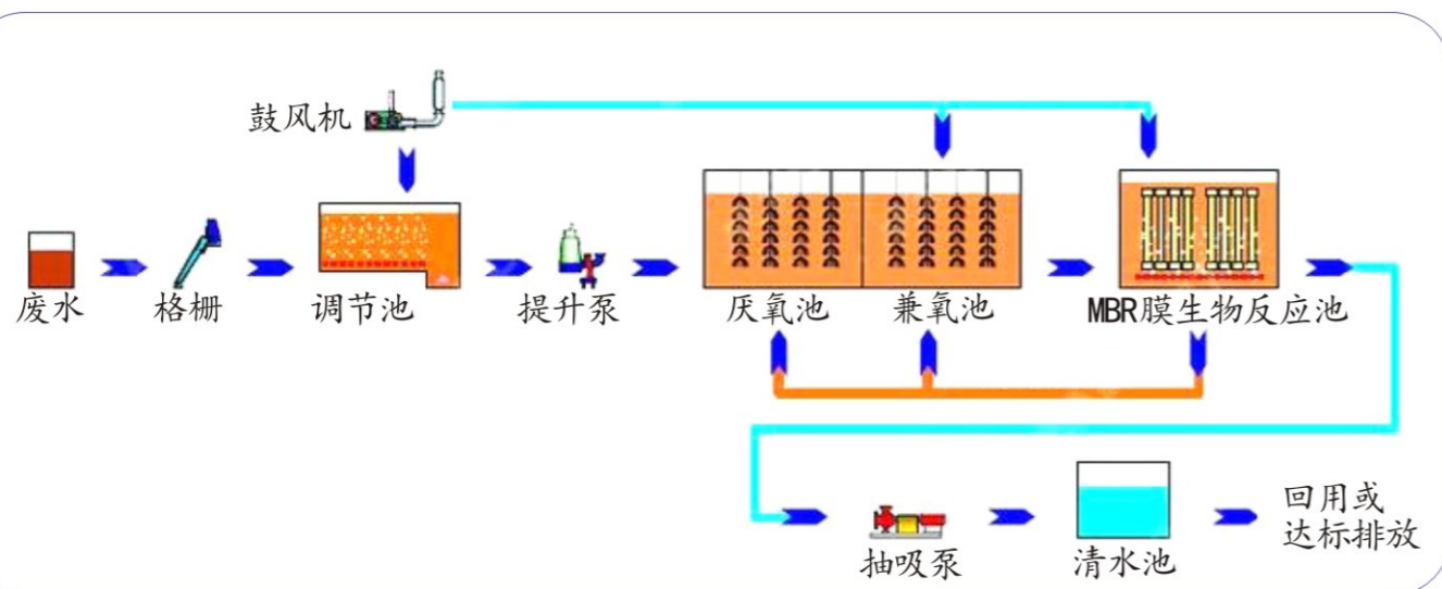
污水处理工艺流程图
