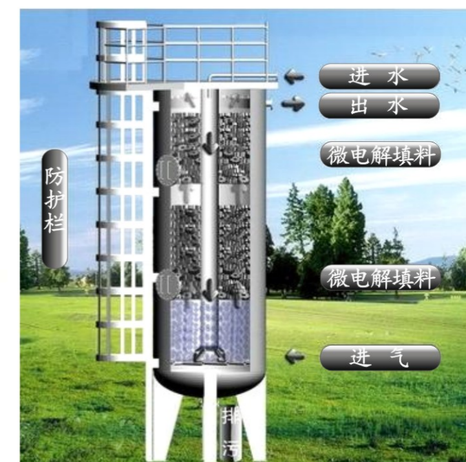
微电解反应工艺流程图
