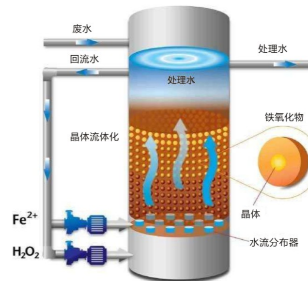
芬顿反应工艺流程图
